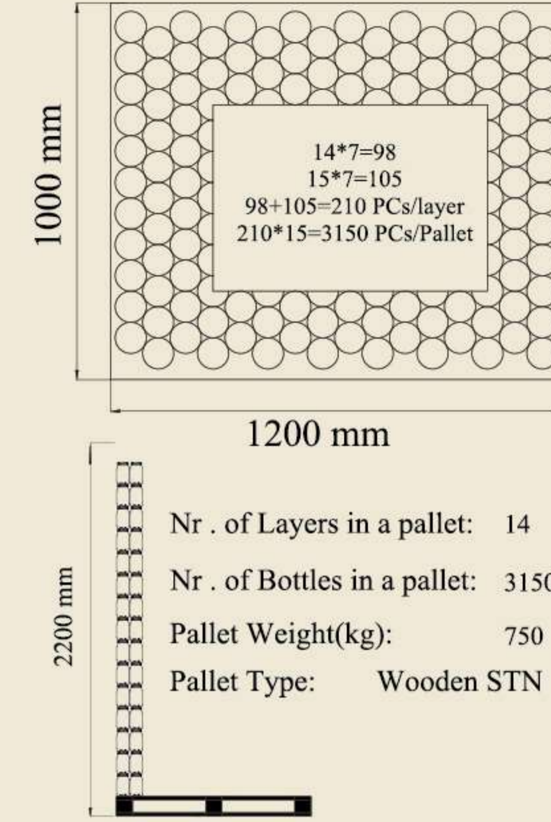
LAYOUT OF BOTTLES IN PALLET چیدمان بطری ها در پالت رسم الزجاجات في البليت
