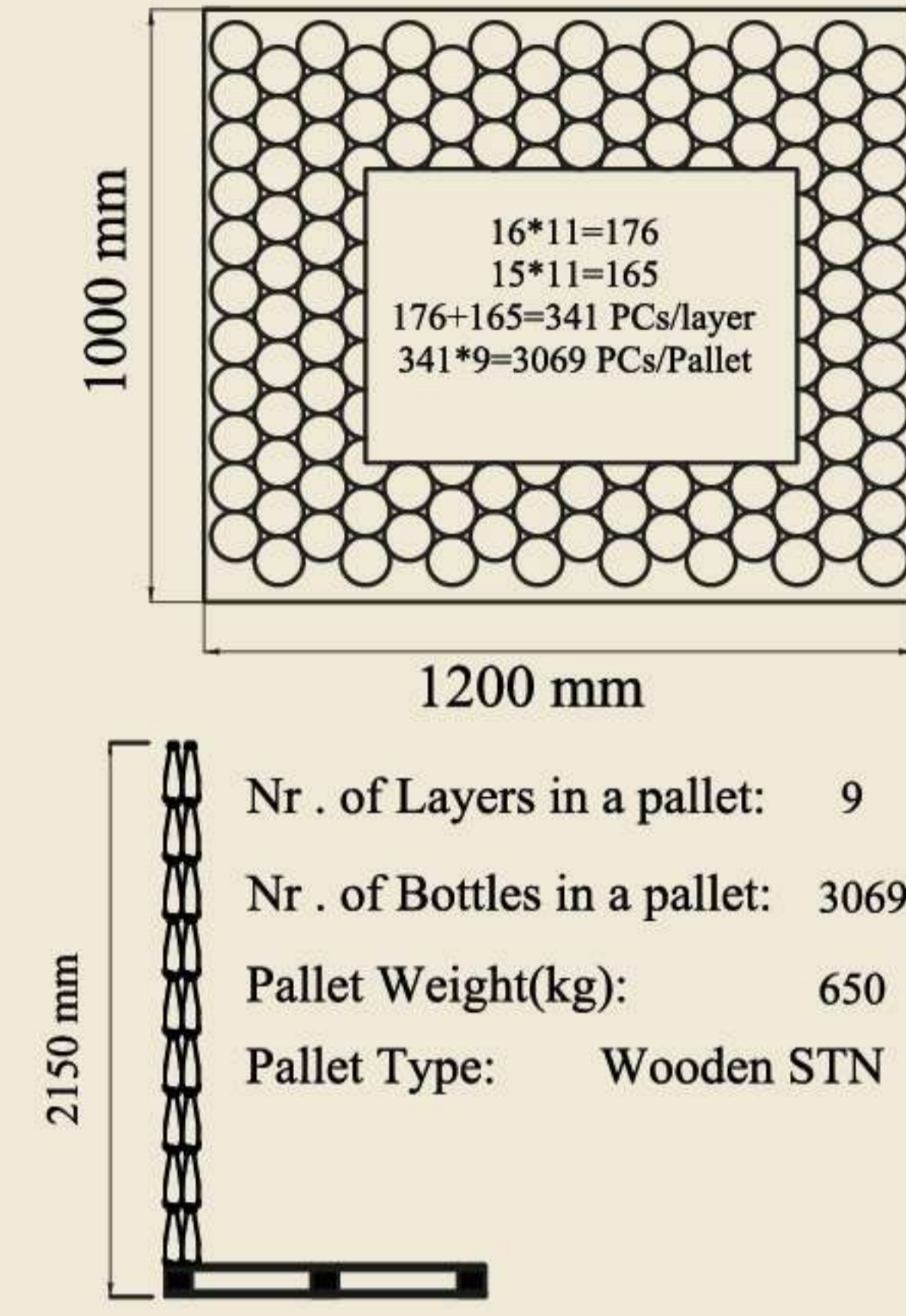
LAYOUT OF BOTTLES IN PALLET چیدمان بطری ها در پالت رسم الزجاجات في البليت
